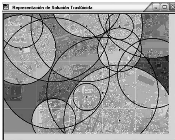
Fig.2 | Simulación de una Topología de red de Telefonía Celular luego de haber considerado 10 generaciones utilizando un AG para optimizar la cobertura en función del tráfico, potencia y zonas prohibidas.
