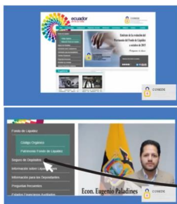
Página web 2016
